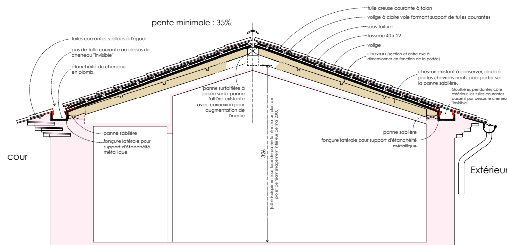
SECTION SUR AILE NORD-OUEST
