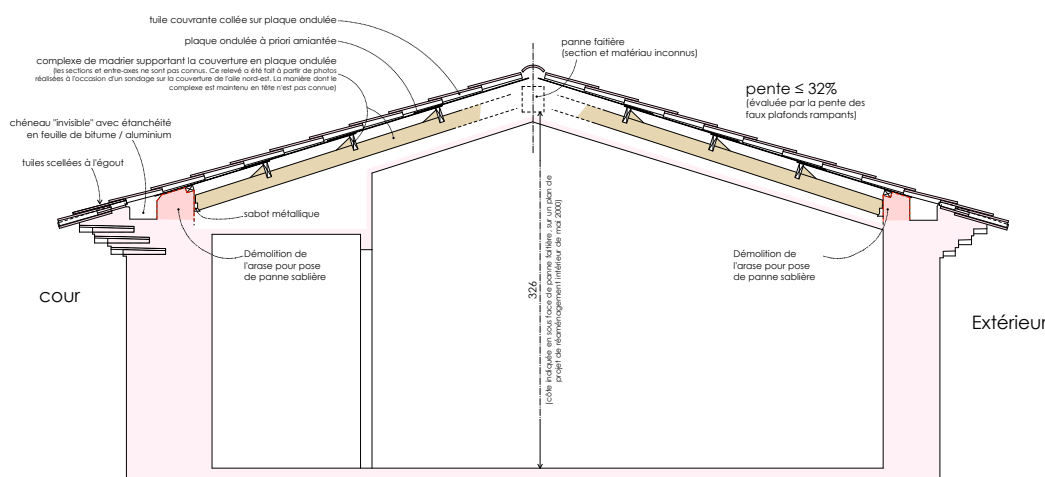
SECTION SUR AILE NORD-OUEST
